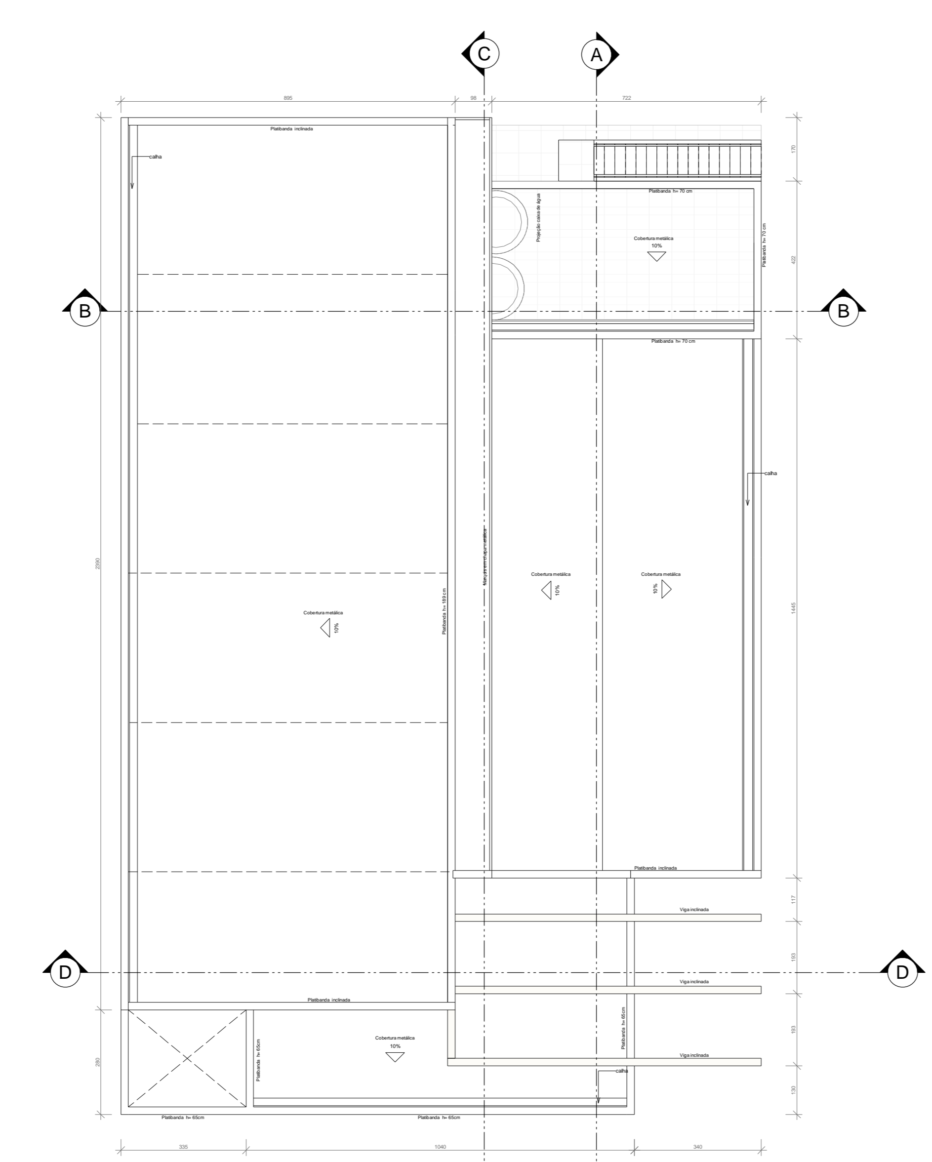
5 COBERTURA ESCALA 1:100
